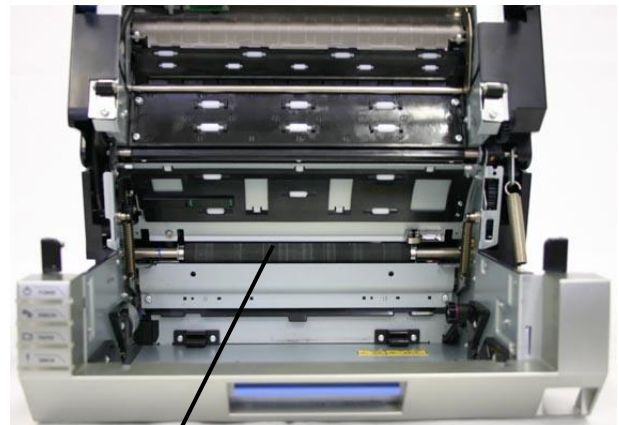
Platen Roller
